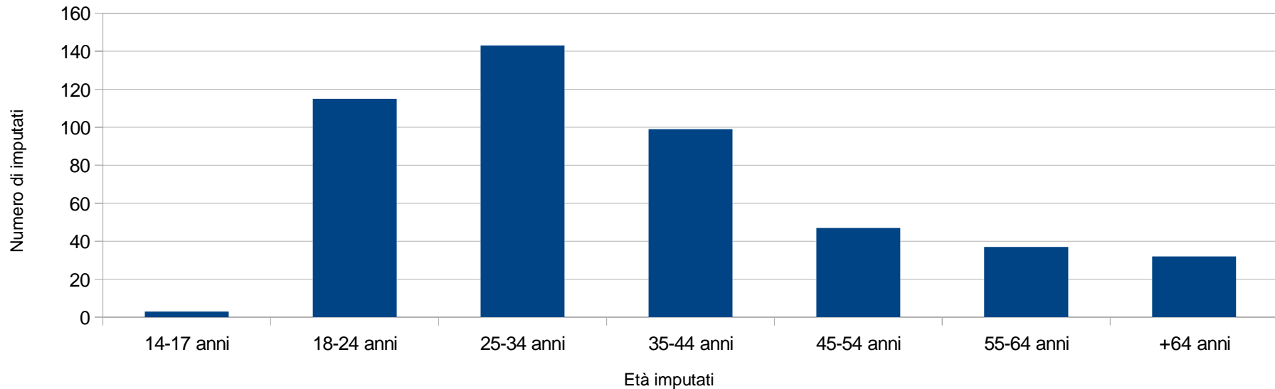
Grafico 2 - Età imputati
