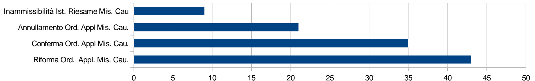
Grafico 6 - Esito Riesame
